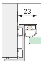
AT 23E Anschlagtürzarge (Eckanschlag, Falzseite)
